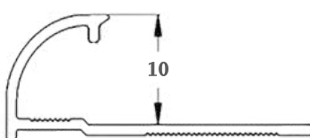
Mã SP: YC10 KT: 10x2500 (mm)
