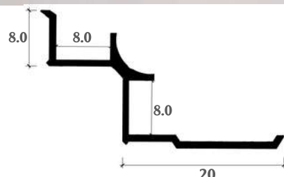
Mã SP: MC8.0 KT: 8x2500 (mm)
