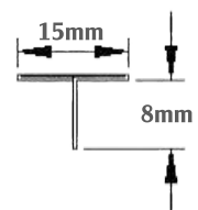
Mã SP: T15
