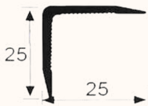
Mã SP: V25 KT: 25x25x2500 (mm)
