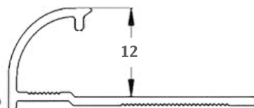
Mã SP: YC12 KT: 12x2500 (mm)
