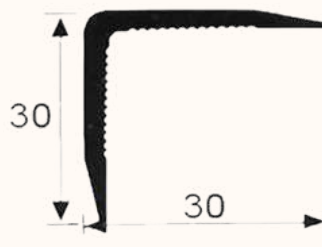
Mã SP: V30 KT: 30x30x2500 (mm)
