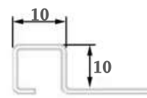
Mã SP: YV10 KT: 10x2500 (mm)
