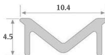
Mã SP: VM10 KT: 10x4.5x2500 (mm)
