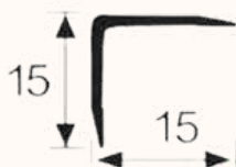
Mã SP: V15 KT: 15x15x2500 (mm)
